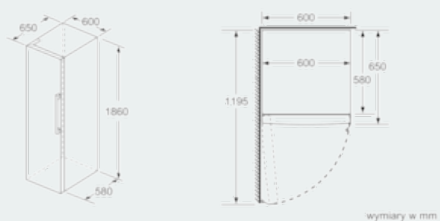
Rysunki wymiarowe
