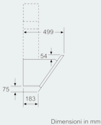
Apparecchio in modalità ricircolo senza canale necessario set per ricircolo Dimensioni in mm
