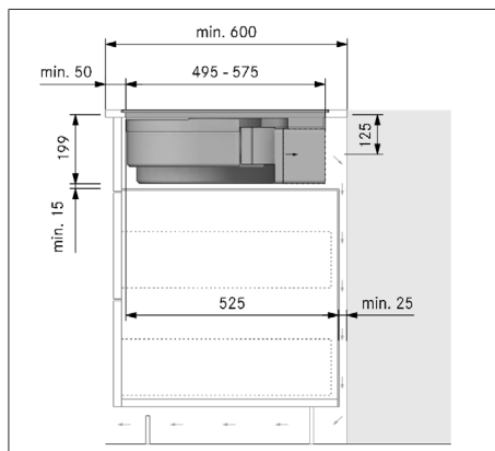
Rys. 11.18 Wymiary zabudowy przy pracy w obiegu zamkniętym – wariant montażowy B, głębokość blatu 600 mm
