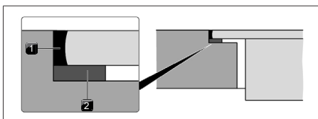
Rys. 11.20 Taśma uszczelniająca przy montażu z zachowaniem równej powierzchni
