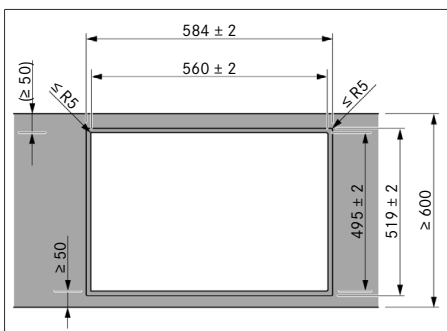
Rys. 11.9 Wymiary wycięcia dla montażu z zachowaniem równej powierzchni
