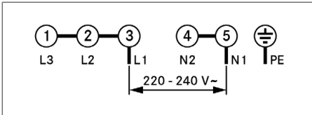
Rys. 11.31 Schemat połączenia – połączenie jednofazowe
