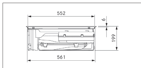
Rys. 3.5 Widok z przodu PURSU2/R
