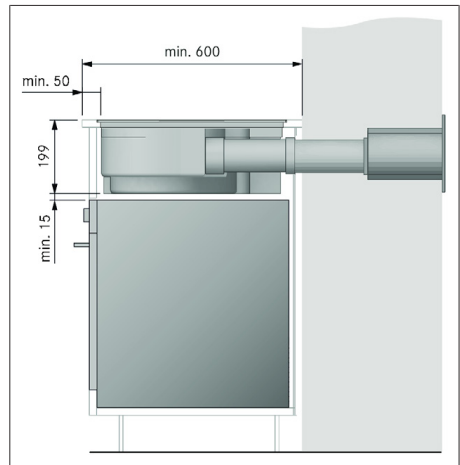
Rys. 11.5 PURSA2/R nad piekarnikiem z prowadzeniem powietrza prosto do tyłu w przejściu ściennym
