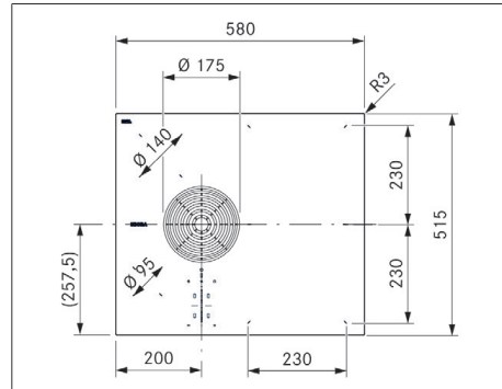
Rys. 3.1 Widok z góry PURSA2/R
