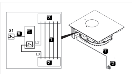
Rys. 11.33 Schemat połączeń z zewnętrznymi stykami przełączającymi
