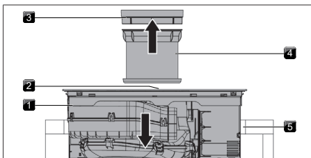
Rys. 11.21 Wkładanie płyty grzewczej
