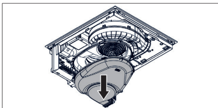
Rys. 11.28 Demontaż dolnej części komory ssawnej
