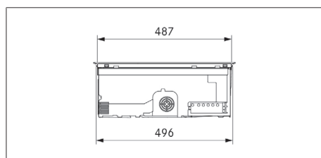
Rys. 3.6 Widok z boku PURSU2/R
