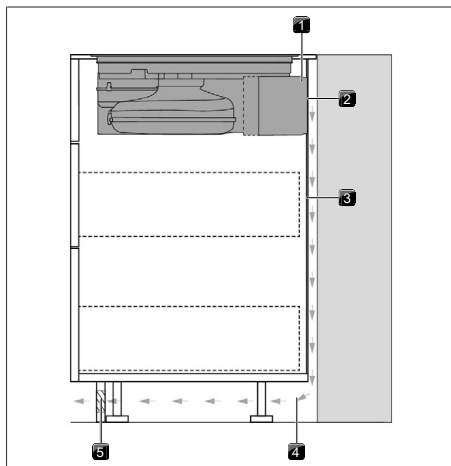
Rys. 11.13 Wariant montażowy z ciągną ścianą tylną
