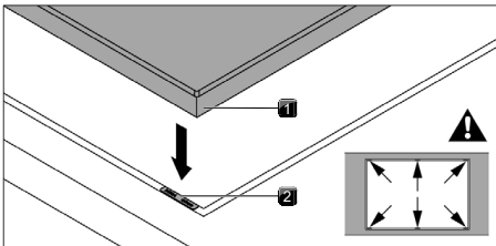
Rys. 11.23 Umieszczenie podkładek wyrównujących
