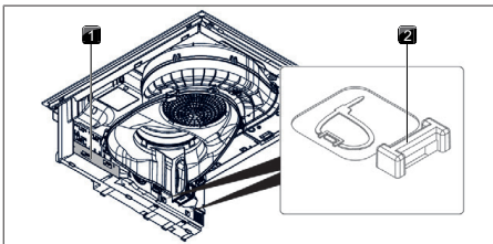
Rys. 11.32 Przyłącza elektryczne płyty grzewczej
