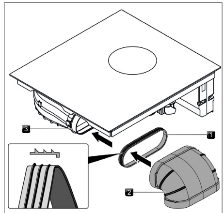
Rys. 11.25 Podłączenie do systemu kanałów
