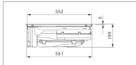
Rys. 3.2 Widok z przodu PURSA2/R
