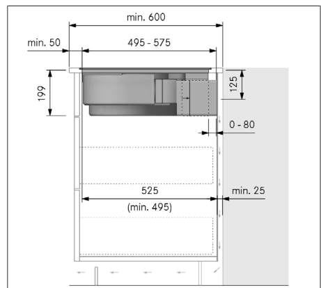
Rys. 11.17 Wymiary zabudowy przy pracy w obiegu zamkniętym, wariant montażowy A
