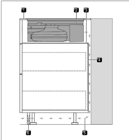
Rys. 11.14 Warianty montażowe z płytą pośrednią
