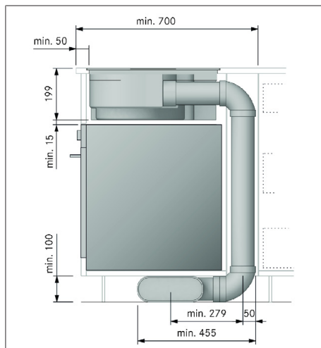
Rys. 11.6 PURSA2/R nad piekarnikiem z przewodzeniem kanału w obszarze cokołu
