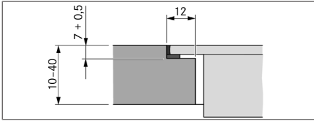
Rys. 11.10 Wielkość zakładki przy montażu z zachowaniem równej powierzchni
