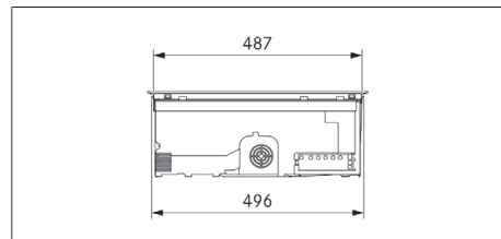
Rys. 3.3 Widok z boku PURSA2/R
