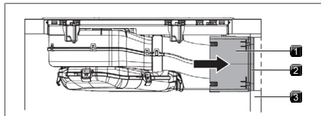
Rys. 11.26 Połączenie z tylną ścianą
