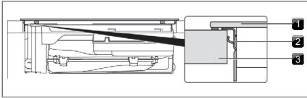
Rys. 11.22 Centralne mocowanie płyty grzewczej
