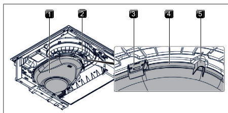
Rys. 9.3 Obudowa kanału powietrza
