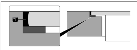
Rys. 11.39 Masa silikonowa przy montażu z zachowaniem równej powierzchni
