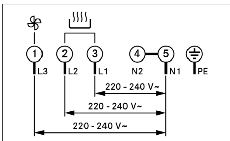
Rys. 11.29 Schemat połączenia – połączenie trójfazowe
