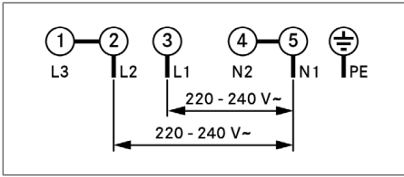
Rys. 11.30 Schemat połączenia – połączenie dwufazowe
