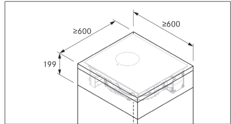
Rys. 11.4 Minimalne wymiary mebli dla S Pure
