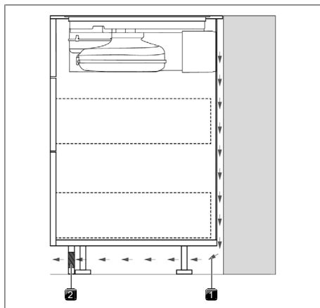
Rys. 11.12 Otwór na strumień zwrotny w obszarze cokołu
