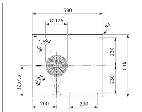
Rys. 3.4 Widok z góry PURSU2/R
