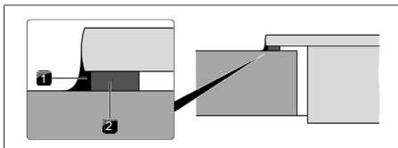
Rys. 11.19 Taśma uszczelniająca przy montażu elementu z uskokiem
