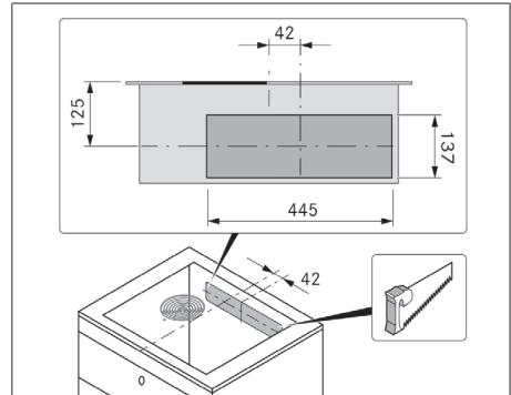
Rys. 11.15 Wycięcie tylnej ściany
