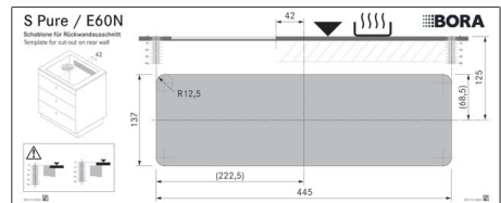
Rys. 11.16 Szablon do wycięcia tylnej ściany
