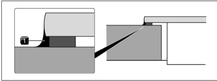
Rys. 11.38 Masa silikonowa przy montażu elementu z uskokiem
