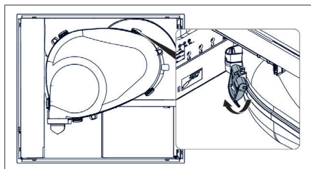
Rys. 11.27 Zamknięcia komory ssawnej
