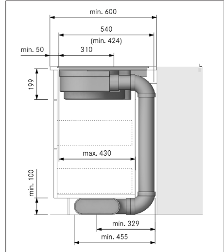
Rys. 11.11 Wymiary zabudowy w przypadku trybu pracy z odprowadzaniem powietrza na zewnątrz, głębokość blatu 600 mm
