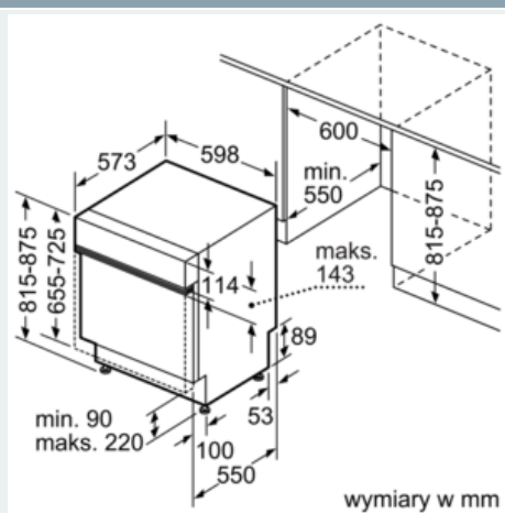
Rysunki wymiarowe
