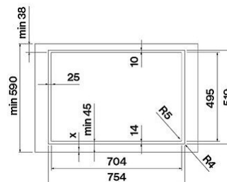
Wymiary otworu
