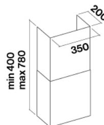
Komin opcjonalny
